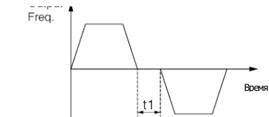
Рис. F1-7. Время перемещения вперед/назад и зона нечувствительности
