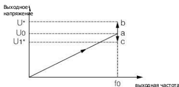
Рис. F5.4. Режим управления напряжением 0 f_0 — заданная частота; U_0 — номинальное напряжение, соответствующее заданной частоте; U^*/U_1^* — установочное значение параметра F5.13 конкретного канала.
